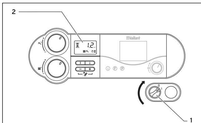
Rys. 4.4 Włączanie kotła
