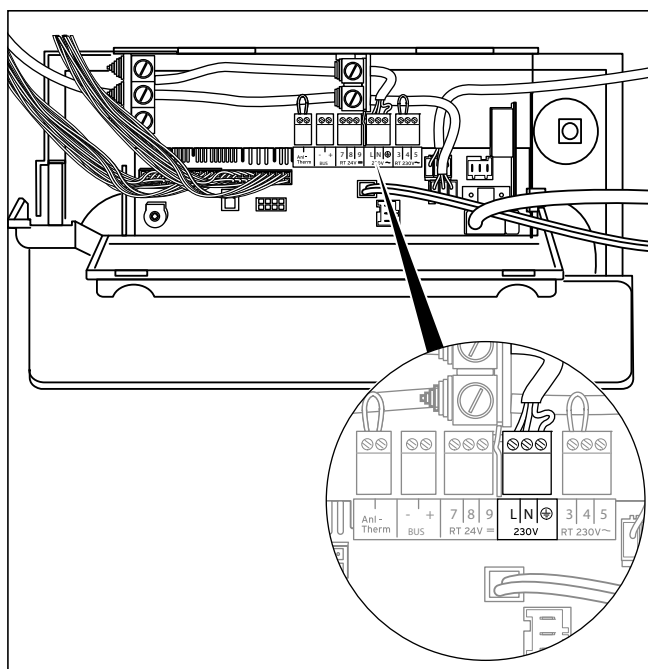
Rys. 5.11 Podłączanie przewodu zasilającego
