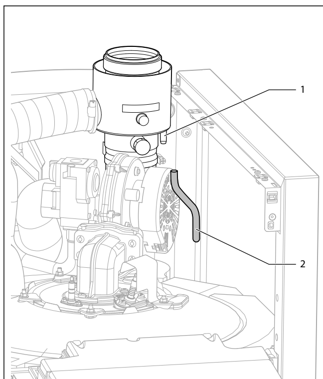
Rys. 8.3 Czyszczenie syfonu
