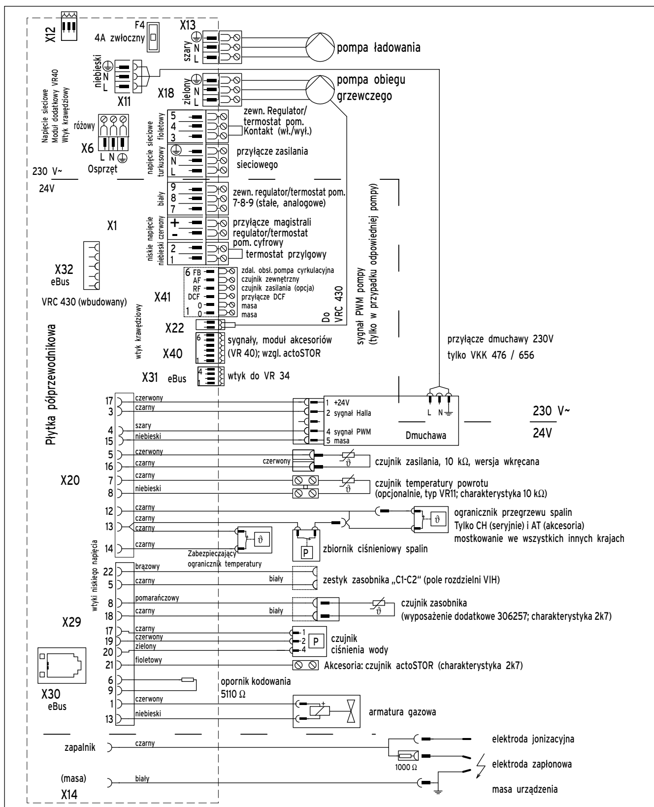
Rys. 5.13 Podłączanie osprzętu elektrycznego okablowania wewnętrznego
