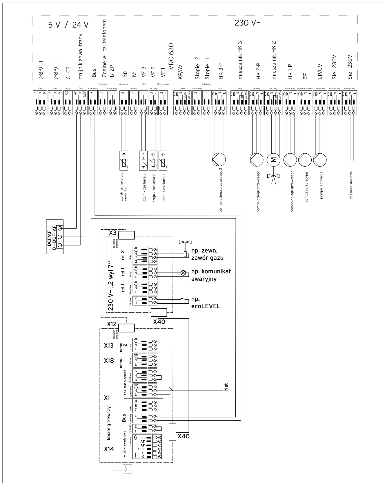
Rys. 5.15 Przyłącze regulatora VRC 620 lub VRC 630
