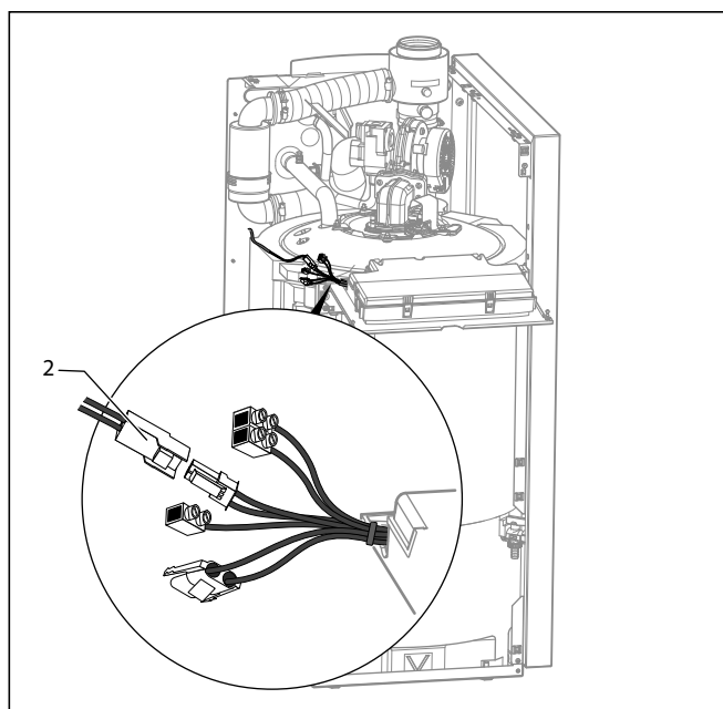
Rys. 5.6 Podłączanie czujnika temperatury zasobnika
