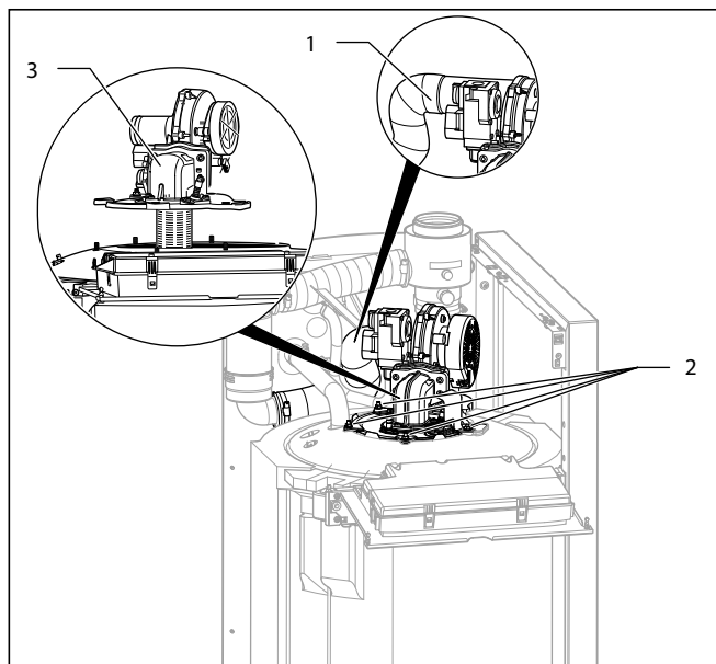
Rys. 8.2 Montaż palnika
