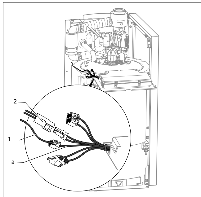
Rys. 5.5 Podłączanie czujnika zasobnika i czujnika temperatury ładowania (actoSTOR)
