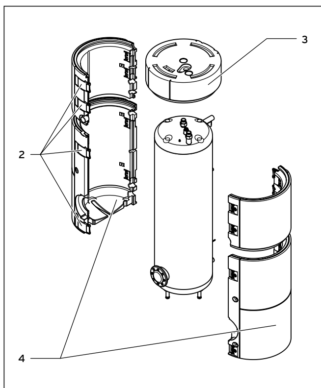
Rys. 5.2 Demontaż izolacji/obudowy
