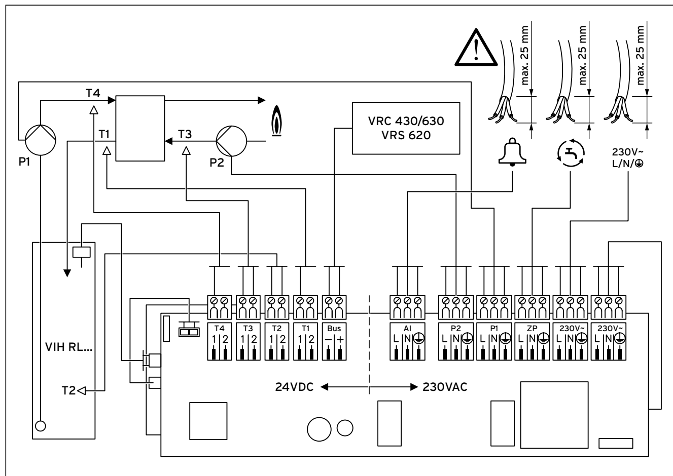
Рис. 5.15 Коммутационная схема
